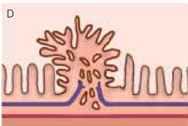
Abb. 3 Adenom-Karzinom-Sequenz
