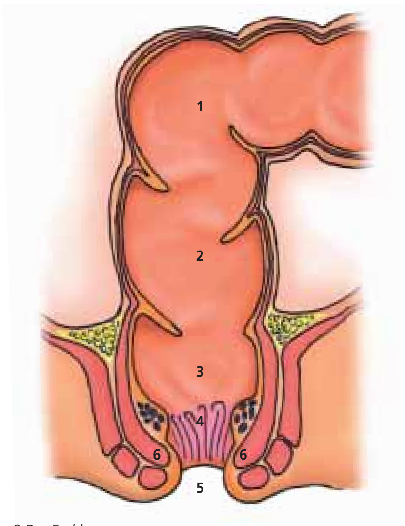
Abb. 2 Der Enddarm
